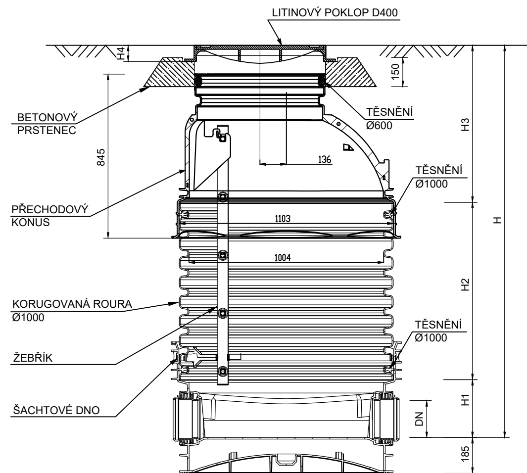
KANALIZAČNÍ ŠACHTA 1000 NG S LITINOVÝM POKLOPEM D400 A S BETONOVÝM PRSTENCEM
